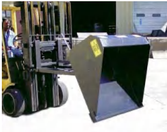
Balde Basculante
